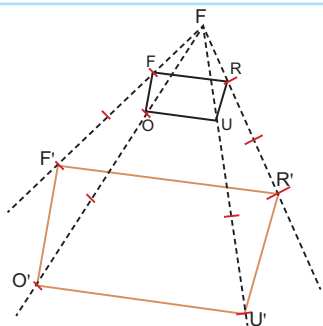
Gambar 4.5 Bangun datar F'O'U'R' didapat dengan cara diperbesar dengan skala 2 dari bangun datar FOUR , maka mereka tidak kongruen
