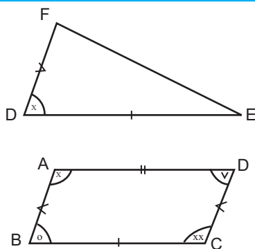
Gambar 4.1 Segitiga DEF dan EFGH tidak kongruen
