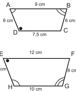
Bangun ABCD dan bangun EFGH sebangun
